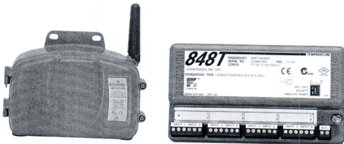
Рисунок 2 - Общий вид преобразователей измерительных Rosemount 848T
