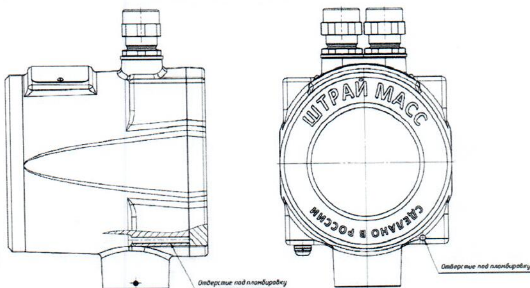
Рисунок 3 – Схема пломбировки ЭБП от несанкционированного доступа счетчиков-расходомеров
