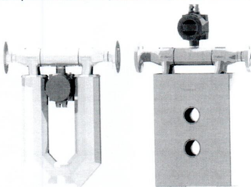
Рисунок 1 – Счётчик-расходомер массовый Штрай-Масс с размещением ЭБП на корпусе ППВ: слева с трубчатым типом кожуха, справа в виде короба
