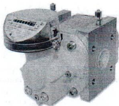
Рисунок 1 - Общий вид счетчика газа
