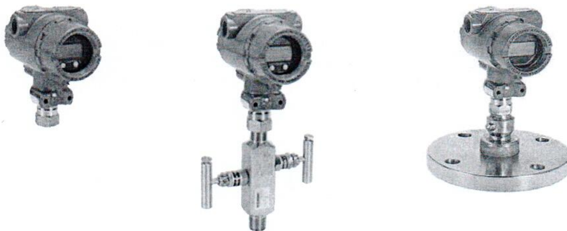
Рисунок 1 – Преобразователи давления измерительные 2088: а) преобразователь 2088; б) преобразователь 2088 в сборе с клапанным блоком 306; в) преобразователь 2088 в сборе с разделительной мембраной 1199
