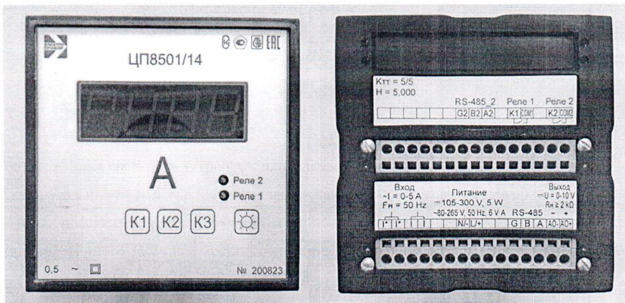
Рисунок 1 – Фотография общего вида устройств с габаритными размерами 120x120x130 мм.
