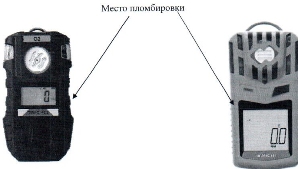
Рисунок 2 - Общий вид газоанализатора ПГ ЭРИС-411-2 и схема пломбировки от несанкционированного доступа
