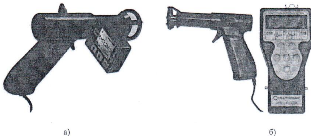
а) ИПС-МГ4.04; б) ИПС-МГ4.01 и ИПС-МГ4.03
