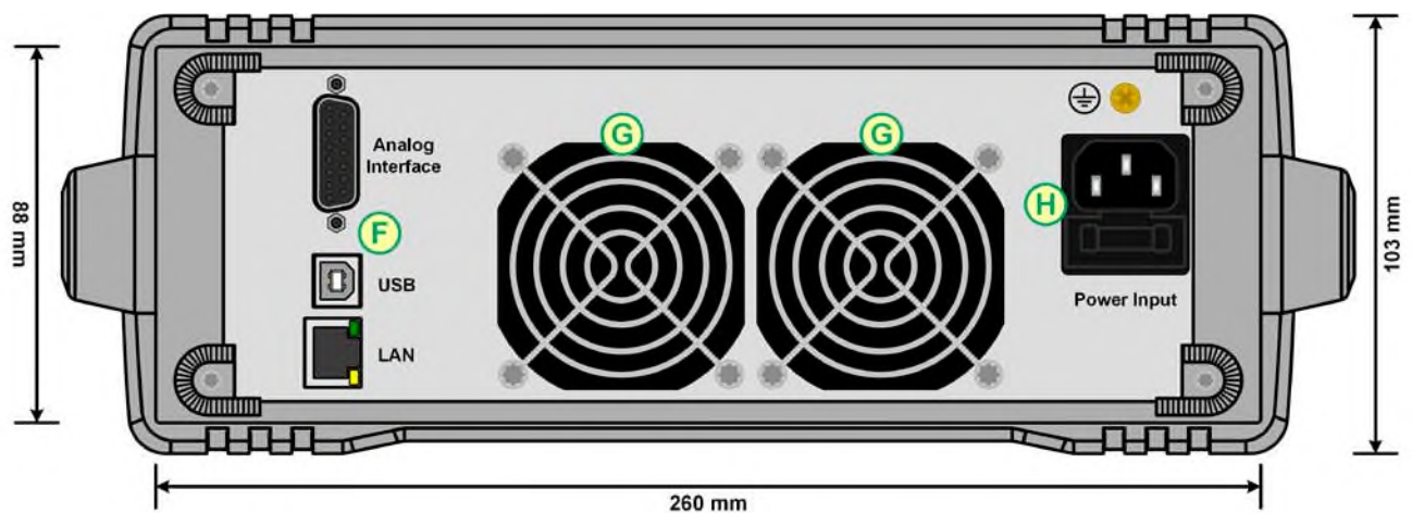
Рисунок 2 - Вид сзади
