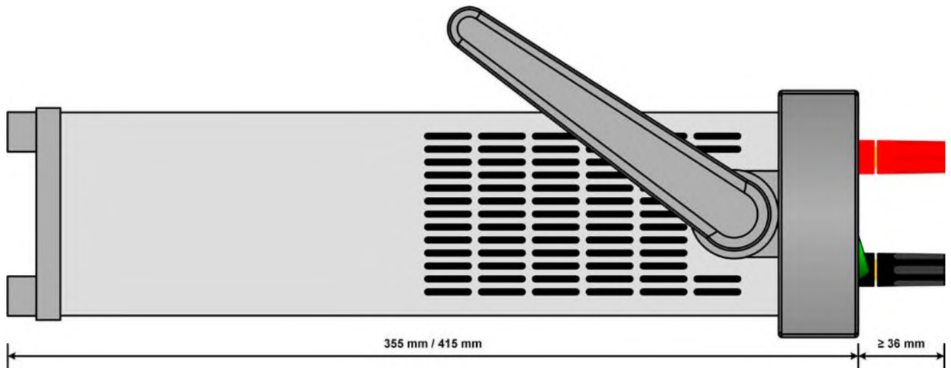
Рисунок 3 - Вид сбоку слева, горизонтальная позиция
