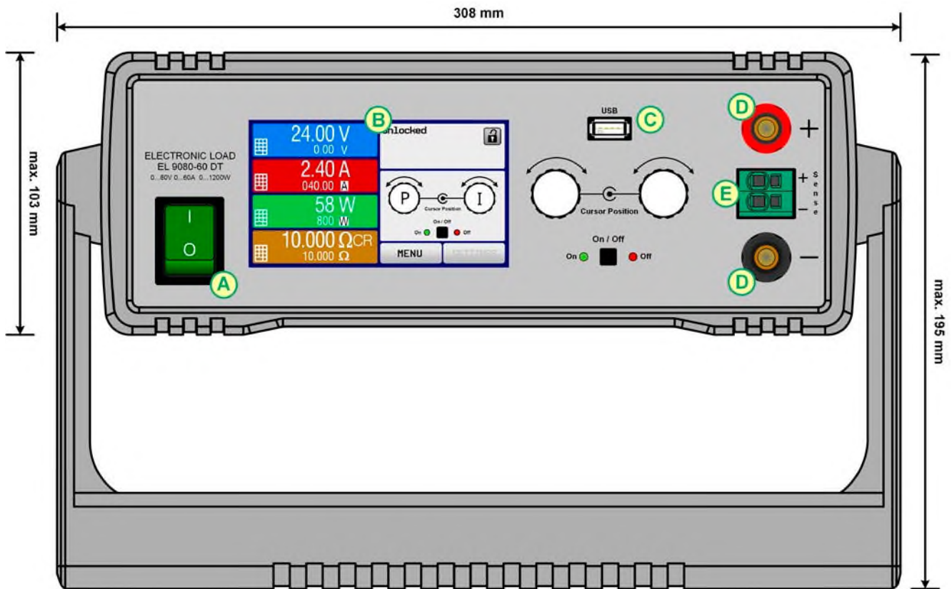
Рисунок 1 - Вид спереди
