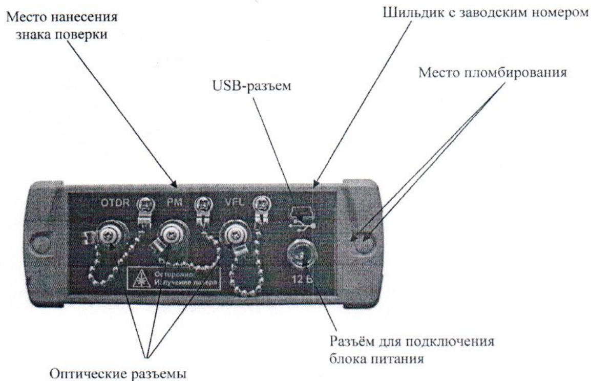
Рисунок 2 - Схема пломбирования и маркировки рефлектометров оптических VISA
