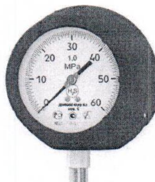
Рисунок 10 – Приборы кислотостойкие
