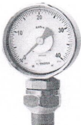
Рисунок 9 – Приборы коррозионностойкие буровые
