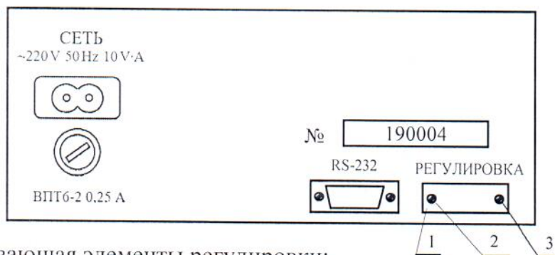
Рисунок А.1 – Схема пломбировки от несанкционированного доступа и указание мест для нанесения оттисков клейм ОТК и поверителя на верхнюю часть корпуса ваттметров
