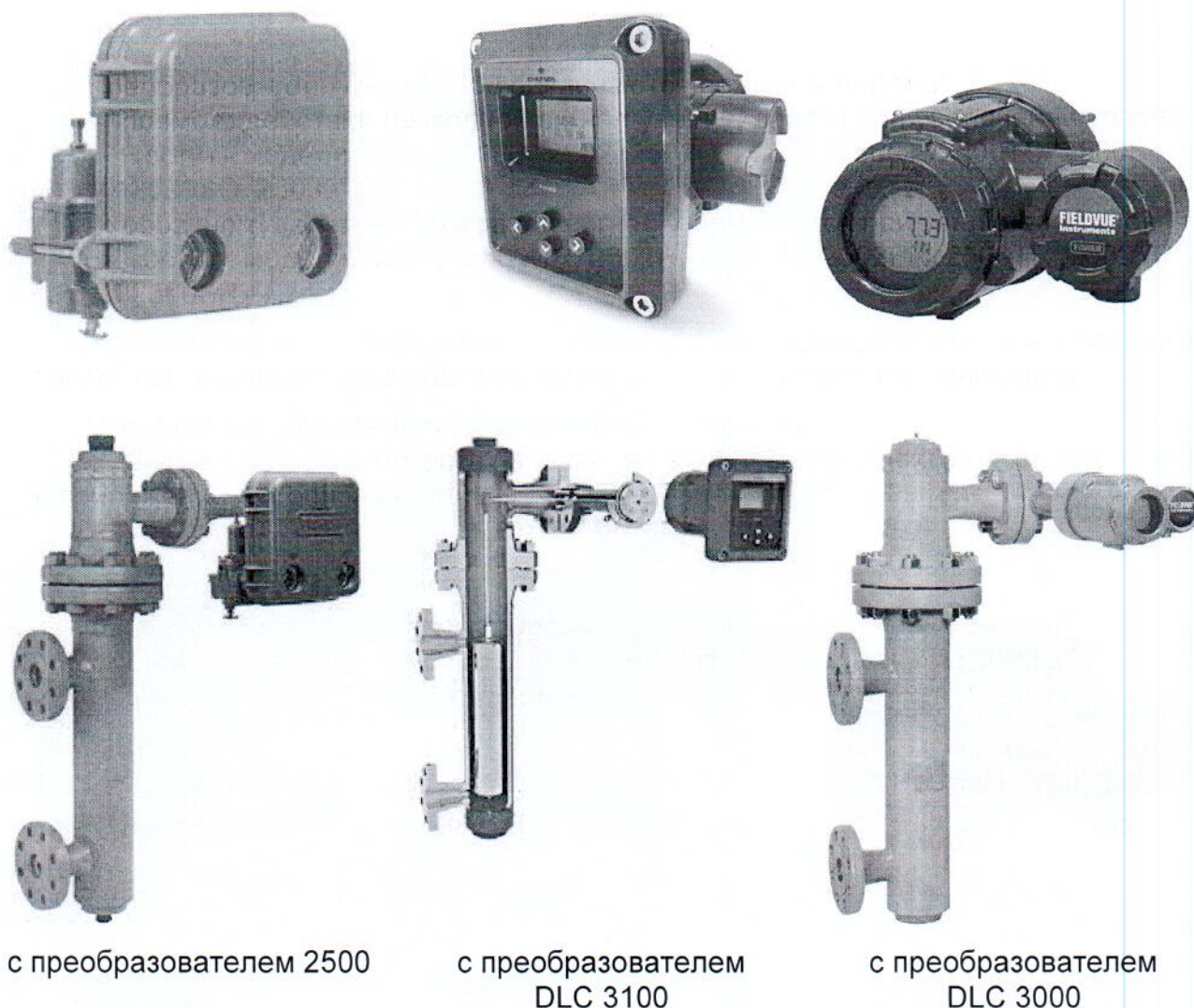
Рисунок 1 – Внешний вид уровнемеров буйковых серии 249 с преобразователями DLC 3xxx и 2500
