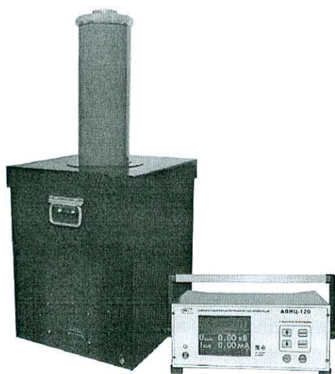
Аппарат высоковольтный испытательный АВИЦ-120
