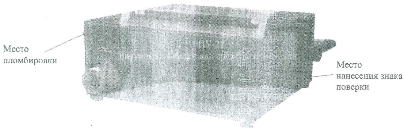
Рисунок 2 - Место пломбировки и место нанесения знака поверки
