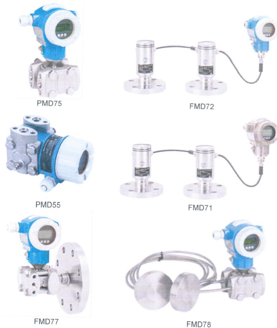
Рисунок 1 – Внешний вид преобразователей дифференциального давления измерительных Deltabar
