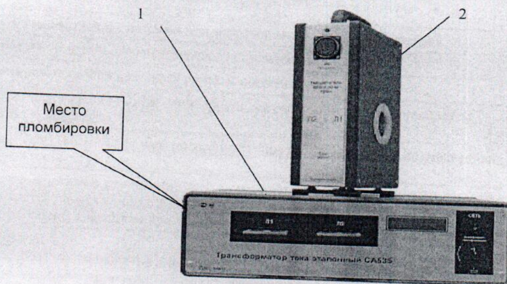
1 - трансформатор СА535, 2- расширитель РД564
