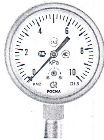
Рисунок 4 – Манометры показывающие KM, KV и KMB в корпусе из нержавеющей стали, серия 22, Кс
