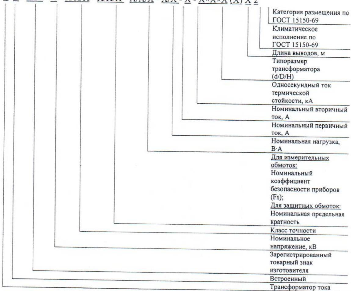
Рисунок 2 - Структура условного обозначения трансформаторов ТВ-НТЗ
