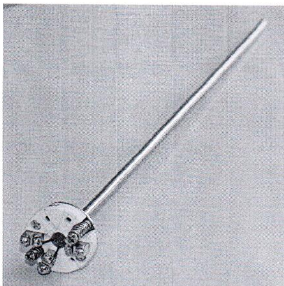
Рисунок 1 – Общий вид термопреобразователей конструктивного исполнения W
