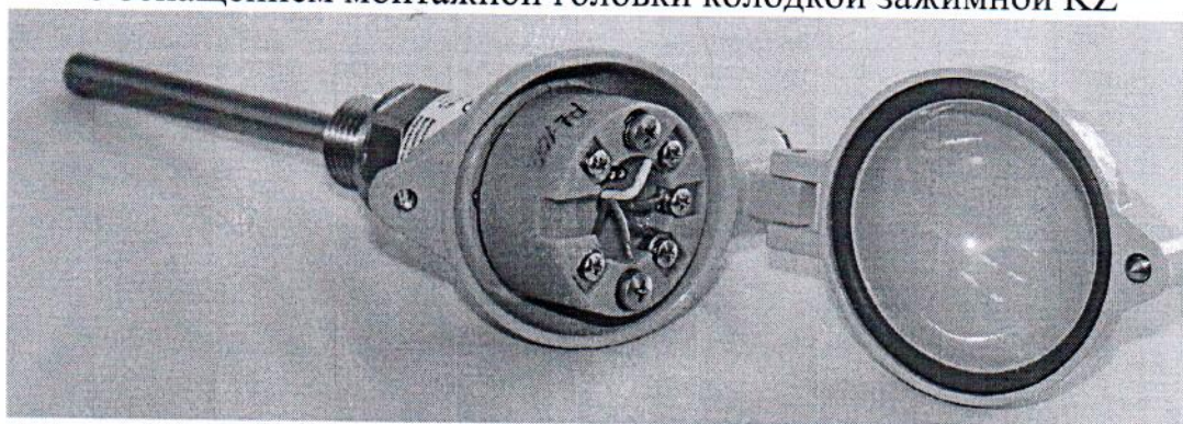
Рисунок 3 – Общий вид термопреобразователей с оснащением монтажной головки преобразователями температуры АТ; АТХ; GI-22; LI-24G; LI-24GX
