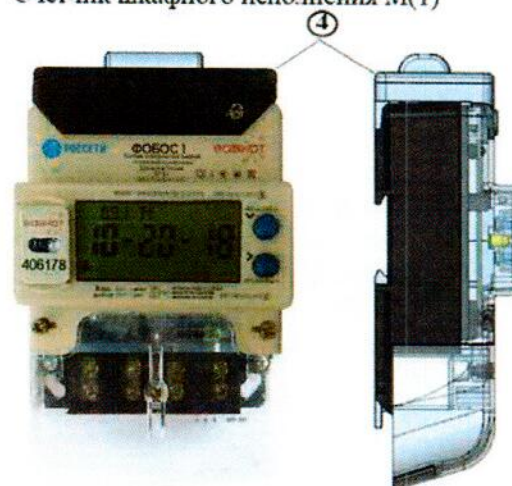
Счетчик шкафного исполнения М(1)
