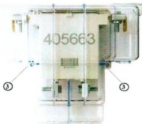
Счетчик «базового» исполнения «Сплит» с клеммными крышками
