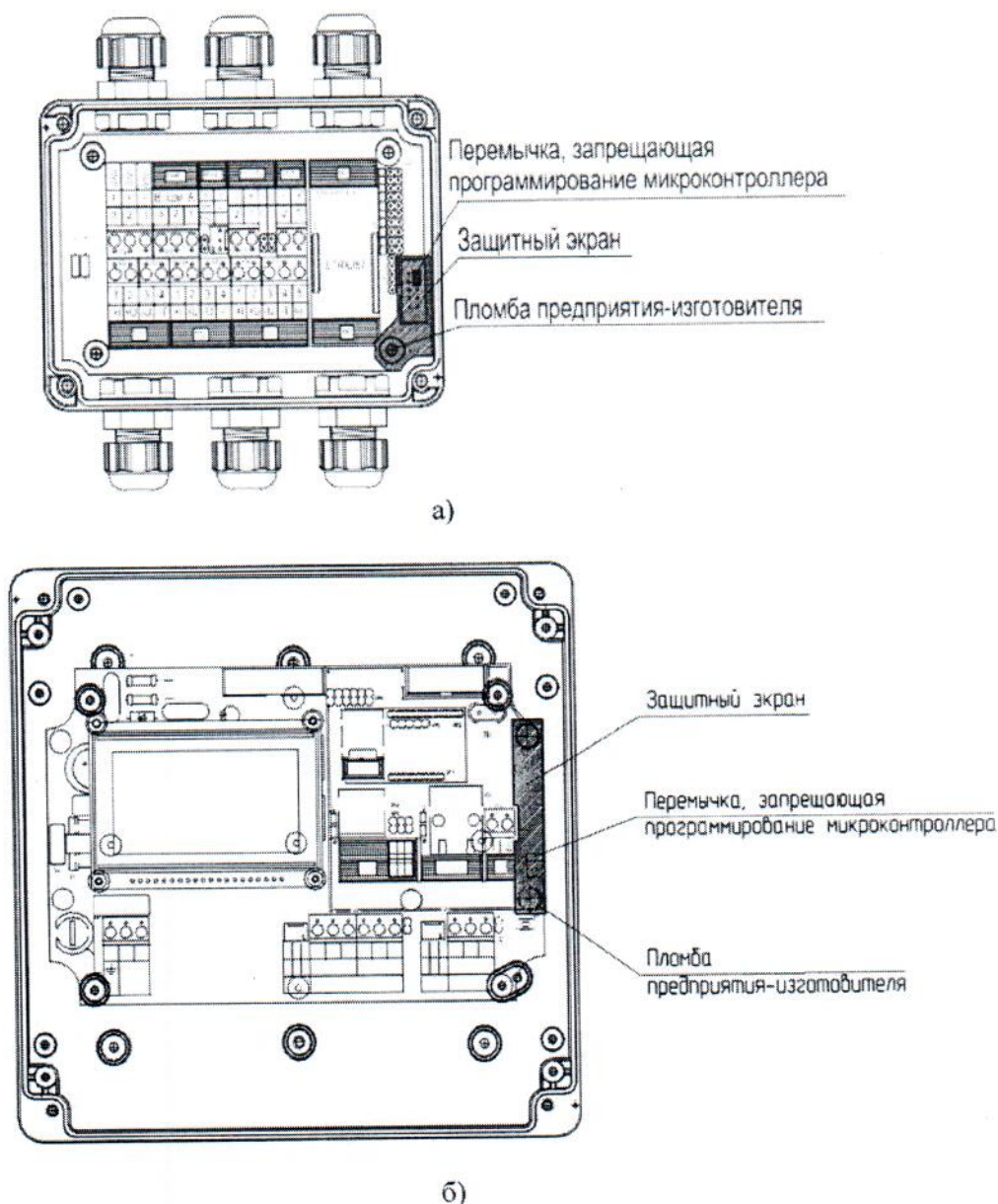
Рис 2. Схемы пломбировки а) ТСМ-ИВП, б) ТСМ-И
