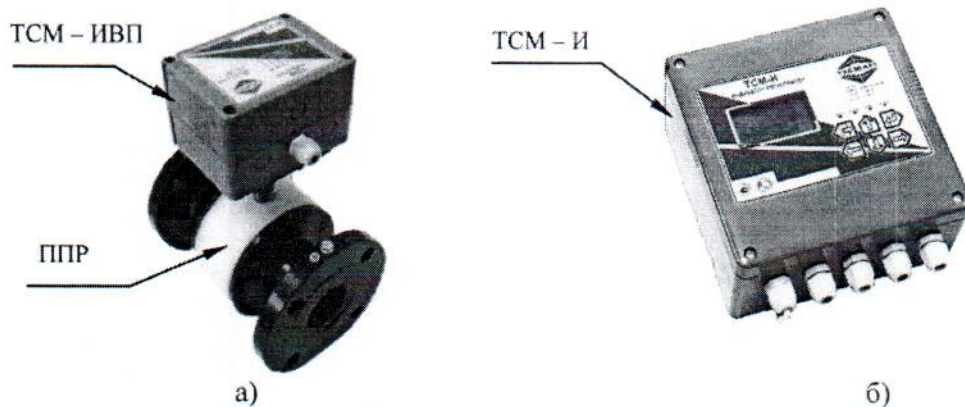
Рис. 1. Теплосчетчик ТСМ
