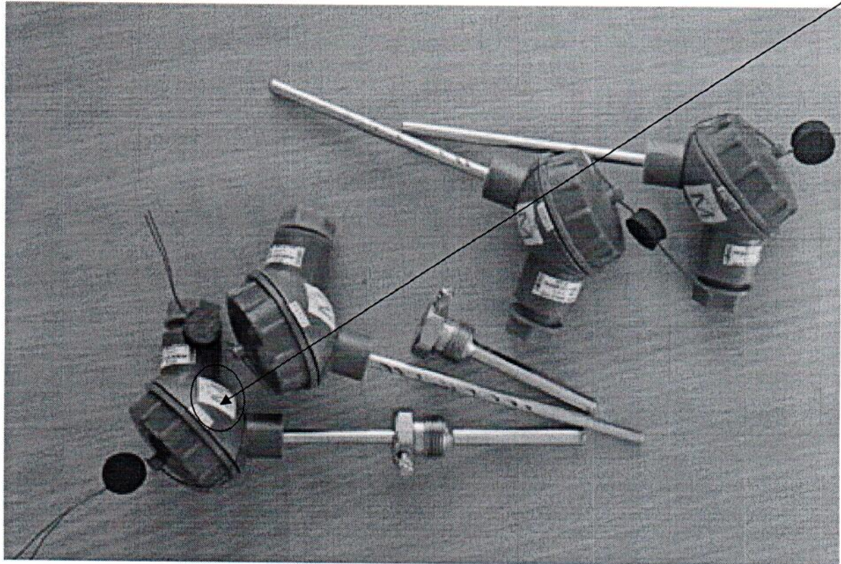
Рисунок А1 - Внешний вид ТС, комплектов ТС и место нанесения знака поверки в виде клейма-наклейки.
