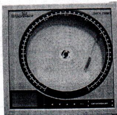
Рисунок 1 – Общий вид ДИСК 250М1
