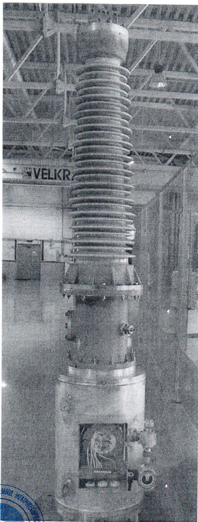
Рисунок 1 - Общий вид трансформаторов напряжения ЗНОГМ
