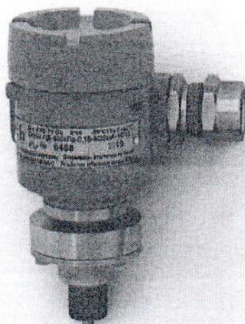
Рисунок 1 – Общий вид преобразователя давления измерительного СЕНС ПД
