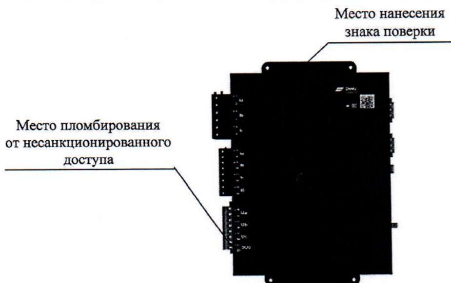
Рисунок 1 – Общий вид устройств ENMU, схема пломбировки от несанкционированного доступа, обозначение места нанесения знака поверки
