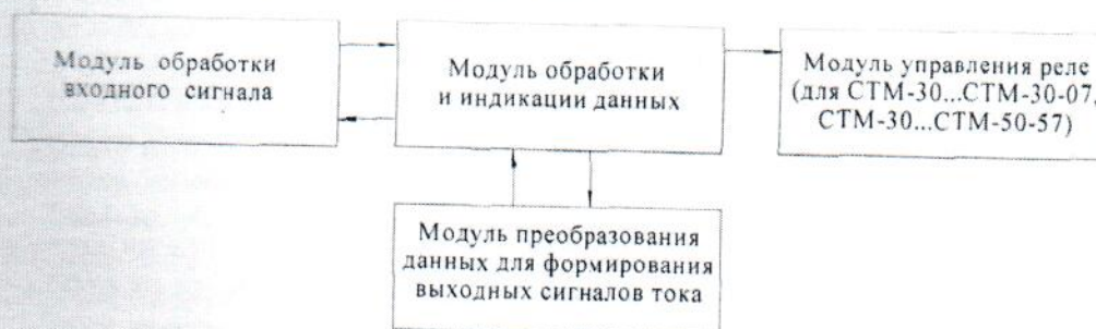
Рисунок 3 – Структура ПО.
