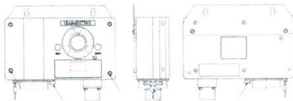
Рисунок 2п - БД сигнализаторов STM-30-10...STM-30-16
