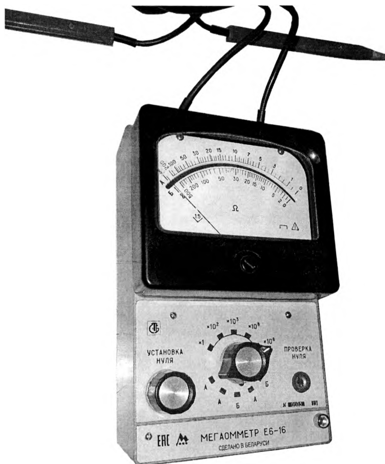
Рисунок 1 – Внешний вид приборов
