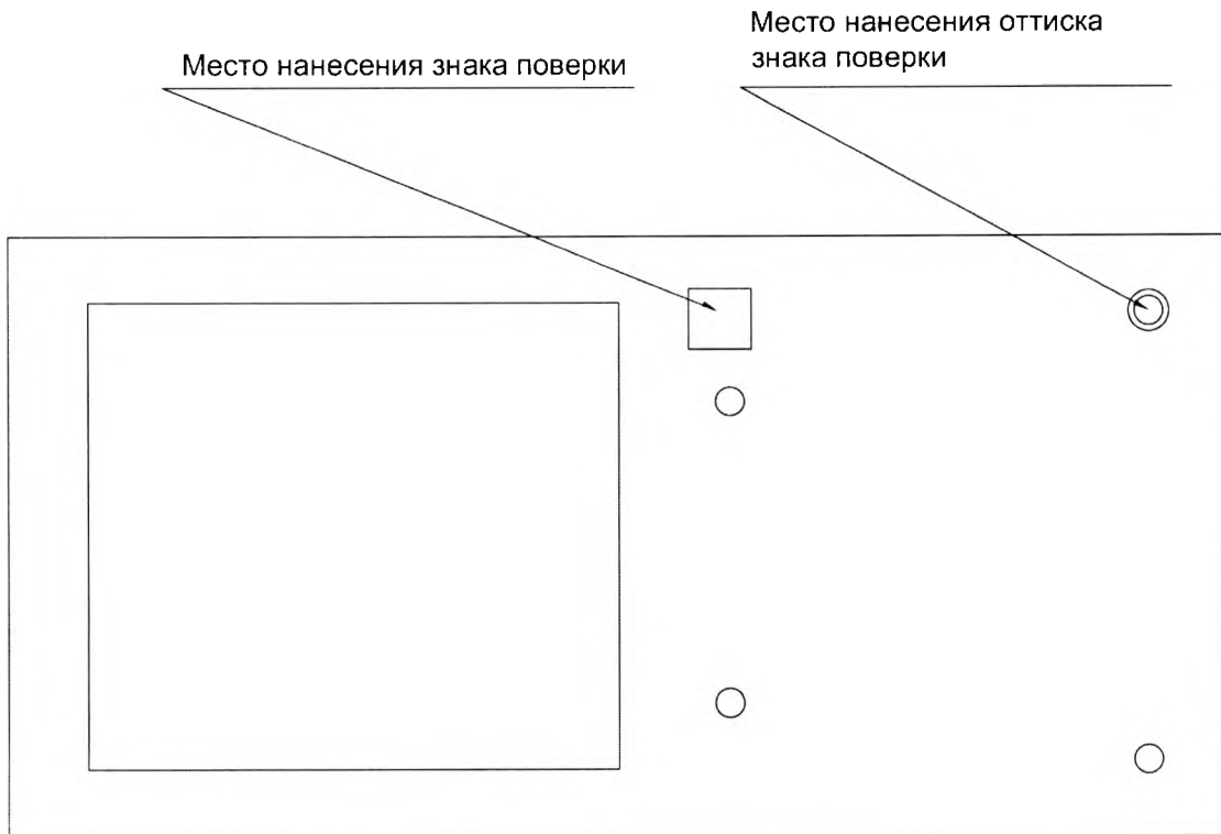
Рисунок А.1 – Верхняя панель мегаомметра Е6-16
