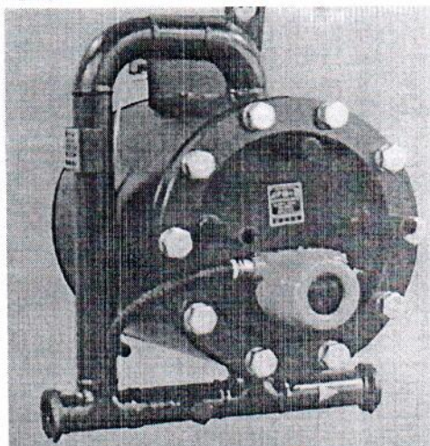
Рисунок 1 - Фотография счетчика жидкости СКЖ обычного исполнения
