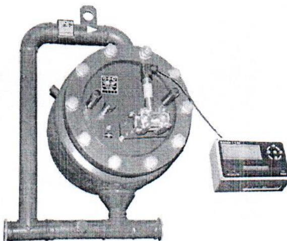
Рисунок 2 - Фотография счетчика жидкости СКЖ точного исполнения
