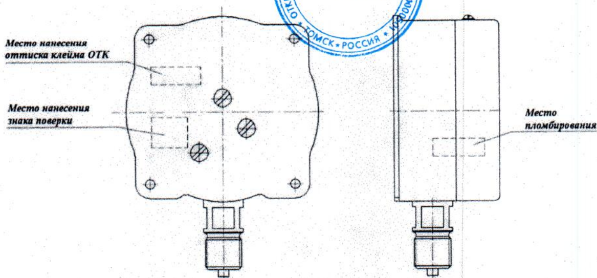
ДА2010Сг вводом ДМ2010Сг, ДВ2010Сг, ДА2010Сг Рисунок 6 - Схема пломбирования от несанкционированного доступа и обозначение мест для нанесения оттисков клейма ОТК и знака поверки
