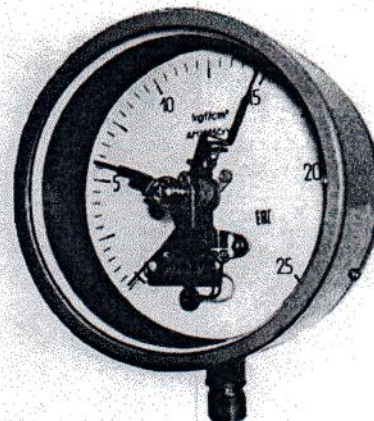
Рисунок 1 - Фотографии общего вида манометров, вакуумметров и мановакуумметров показывающих сигнализирующих ДМ2005Сг, ДВ2005Сг, ДА2005Сг
