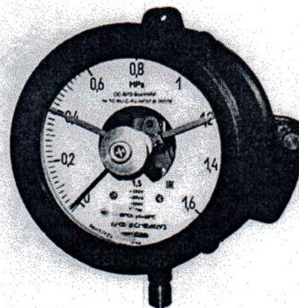
Рисунок 3 - Фотографии общего вида манометров, вакуумметров и мановакуумметров показывающих сигнализирующих ДМ2005Сг1ЕхКс, ДВ2005Сг1ЕхКс, ДА2005Сг1ЕхКс
