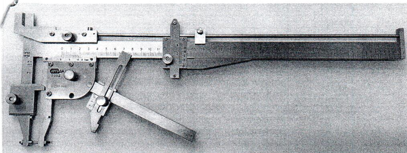
Рисунок 1 – Общий вид штангенциркуля путевого модели ПШВ-01
