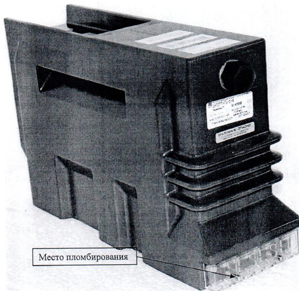
Рисунок 4 – Общий вид трансформаторов комбинированных НТОЛП-НТЗ
