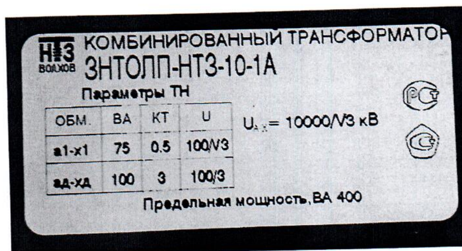
Рисунок 5 – Табличка технических данных трансформаторов комбинированных ЗНТОЛП-НТЗ (параметры трансформатора напряжения)
