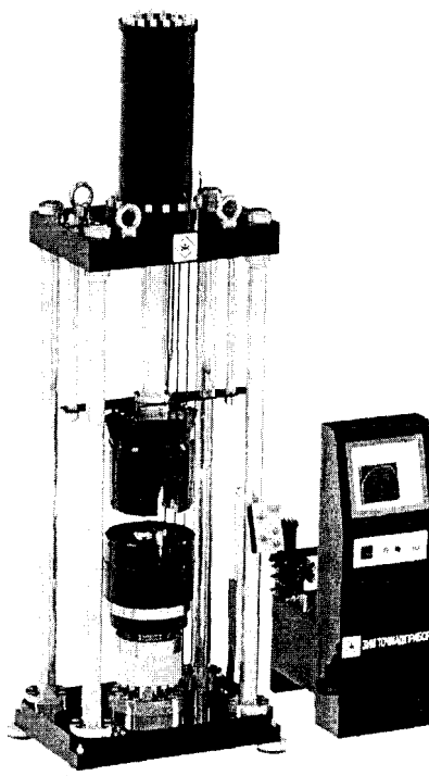
Рисунок 2 - Общий вид машины универсальной испытательной типа ИР-1000-1М Пломбирование машин испытательных универсальных РМ-УМ1 и ИР-1М не предусмотрено.
