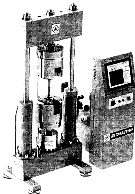
Рисунок 1 - Общий вид машины универсальной испытательной типа РМ-УМ1
