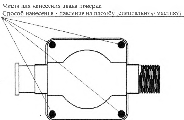
Рисунок 3 - Схема пломбировки от несанкционированного доступа, обозначения места нанесения знака поверки
