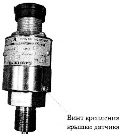
Рисунок 1 - Общий вид преобразователей давления ТП-140Д
