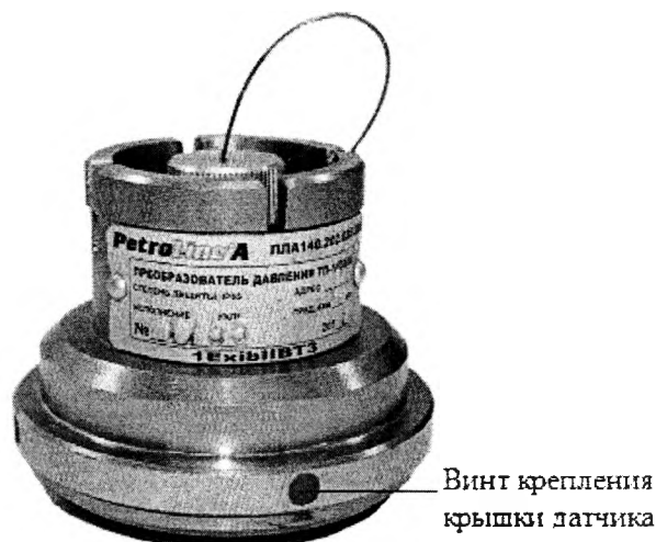
Рисунок 2 - Общий вид преобразователей давления ТП-140Д(М)
