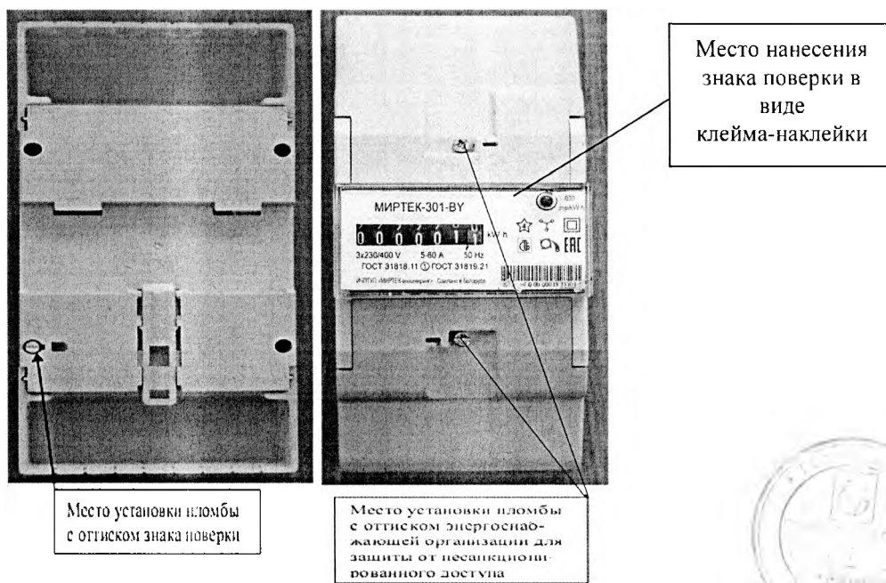
Рисунок А.4 – Места установки пломб и нанесения знака поверки для счетчиков в корпусе модификации D33
