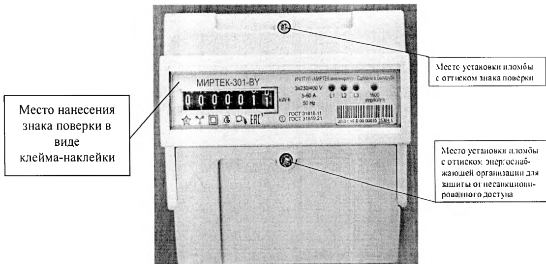
Рисунок А.5 – Места установки пломб и нанесения знака поверки для счетчиков в корпусе модификации D34
