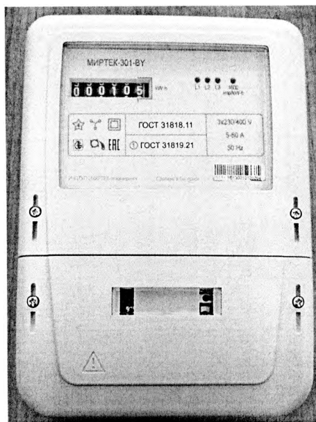
Рисунок 2 – Общий вид счетчика в корпусе модификации W31
