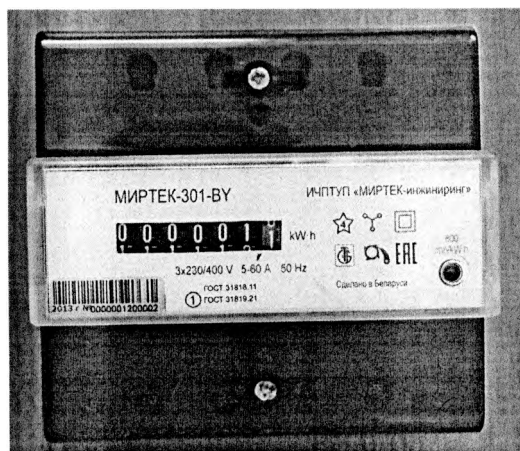
Рисунок 3 – Общий вид счетчика в корпусе модификации D31
