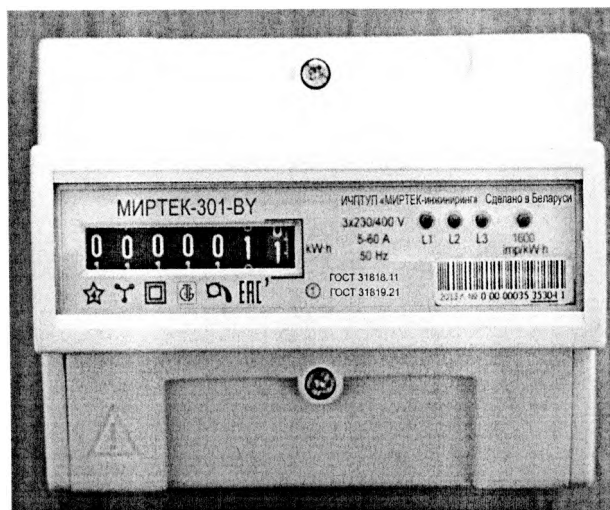
Рисунок 5 – Общий вид счетчика в корпусе модификации D33
