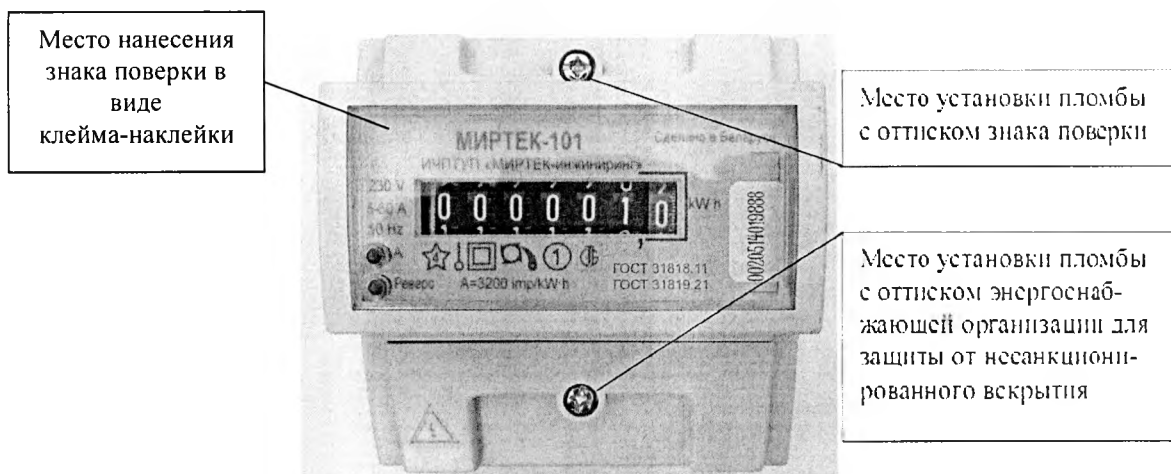
Рисунок А.4 – Места установки пломб и нанесения знака поверки для счетчиков в корпусе модификации D3
