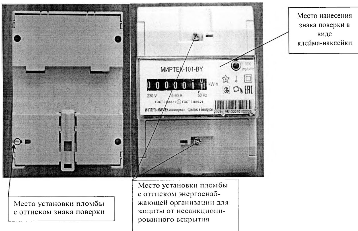
Рисунок А.3 – Места установки пломб и нанесения знака поверки для счетчиков в корпусе модификации D1
