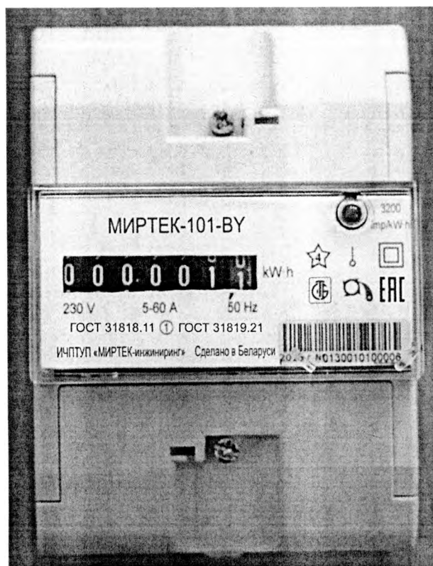
Рисунок 4 – Общий вид счетчика в корпусе модификации D1
