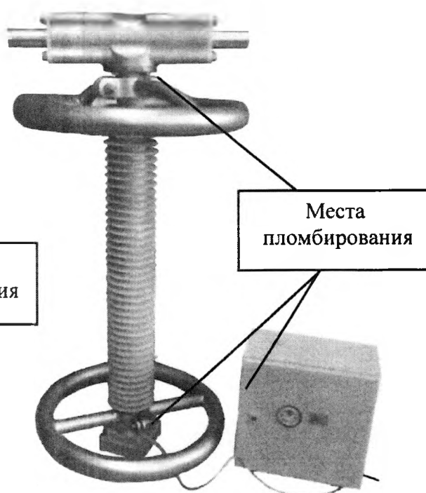
Рисунок 5 - Внешний вид исполнения ЦТТН 35 - 220 кВ опорного исполнения с электронным блоком в отдельном шкафу
