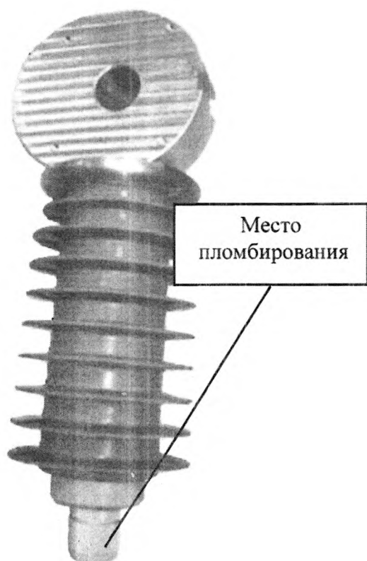
Рисунок 7 - Внешний вид исполнения ЦТН 6(10) -35 кВ подвешного исполнения (электронный блок, выполненный в отдельном корпусе представлен на рисунках 2 и 5)
