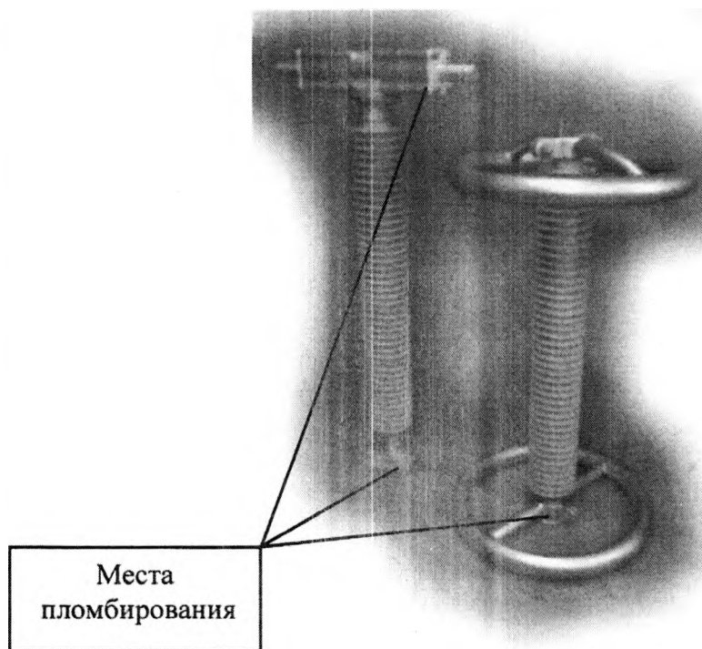
Рисунок 4 - Внешний вид исполнения ЦТТН 35 - 220 кВ опорного исполнения с электронными блоками в голове и основании колонны
