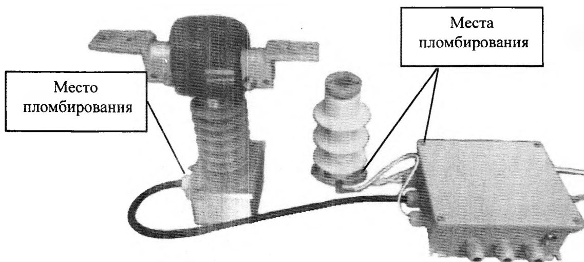
Рисунок 3 - Внешний вид ЦТТН 6(10) -35 кВ опорного исполнения с двумя измерительными узлами для измерения силы тока и напряжения с электронным блоком, выполненным в отдельном корпусе
