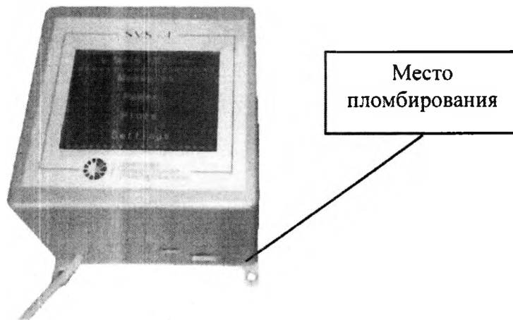
Рисунок 9 - Устройство отображения результатов измерений ЦТН 6(10) -220 кВ
