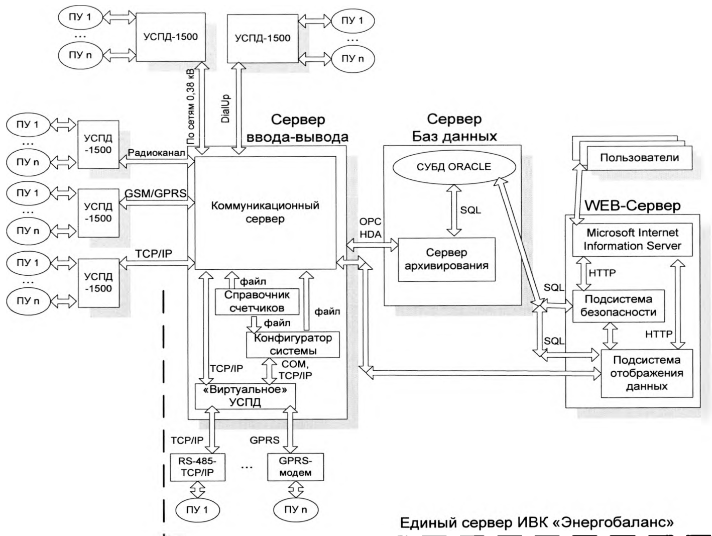
Рисунок 1 – Структурная схема комплексов измерительно-вычислительных для учета энергоресурсов «ЭНЕРГОБАЛАНС».
