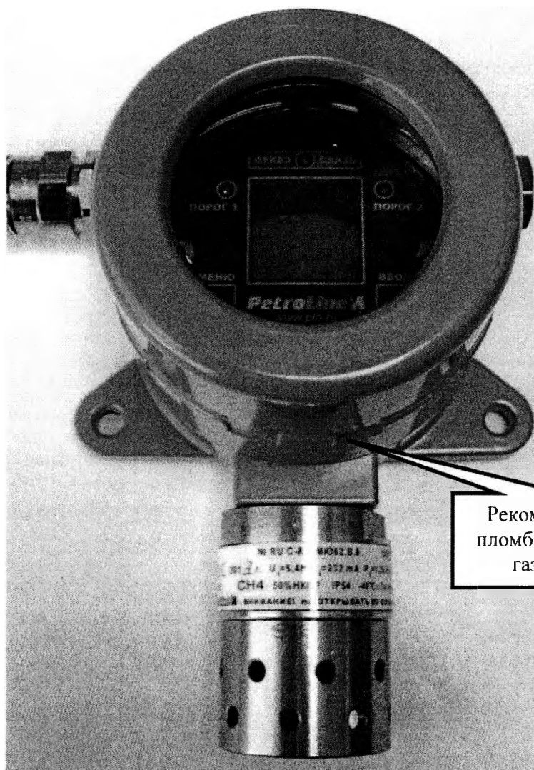
Рисунок 1 - Общий вид газоанализаторов и схема пломбирования корпуса газоанализатора от несанкционированного доступа
