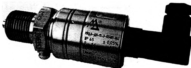
Рисунок 1 - Общий вид датчика давления МИДА-15
