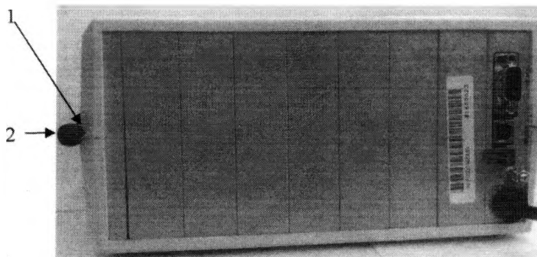
Рисунок 2 – Схема пломбировки от несанкционированного доступа, обозначение места нанесения знака поверки комплексов поверочных «ВЗЛЕТ КПИ»
