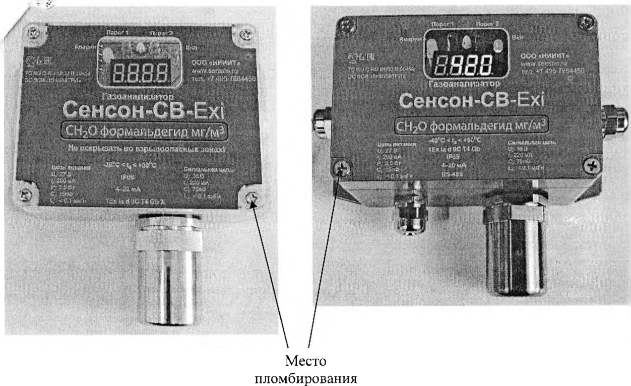
Рисунок 3 - Общий вид исполнения СВ (в пластмассовом или металлическом корпусе)
