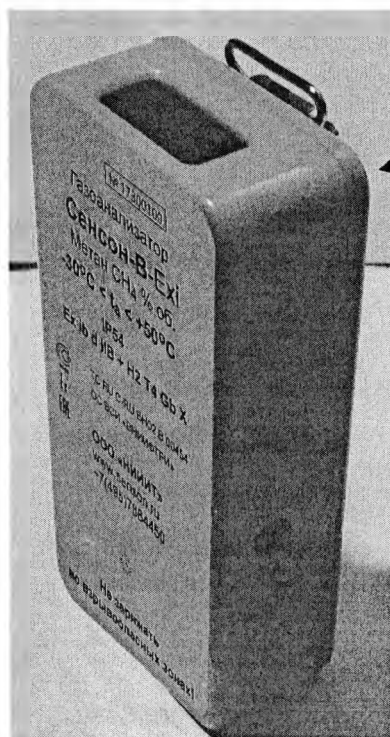
Рисунок 1 - Общий вид исполнения В (индивидуального)
