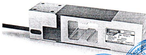
Рисунок 4 – Внешний вид датчиков Т40А
