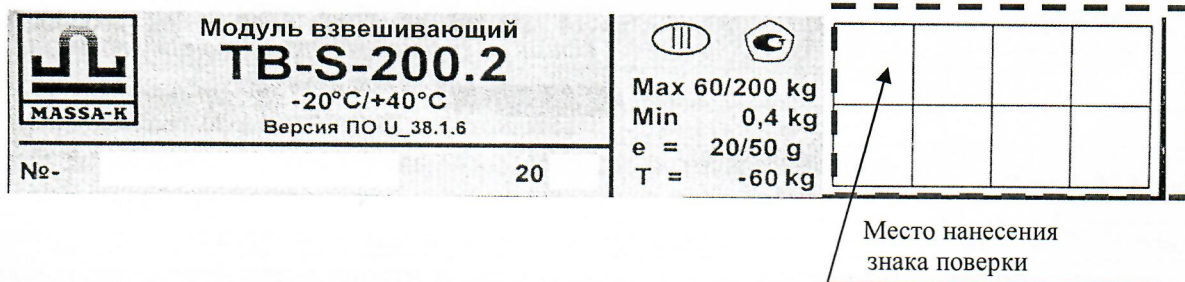
Рисунок 3 – Маркировка и место нанесения знака поверки
