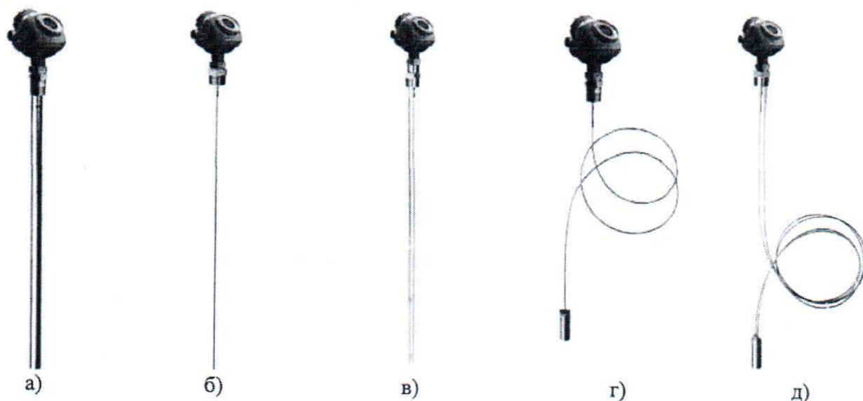
Рисунок 1 - Общий вид уровнемеров 5300 с различными типами волноводов (зондов): а) коаксиальный, б) жесткий одинарный или сегментированный жесткий одинарный, в) жесткий двойной, г) гибкий одинарный с грузом, д) гибкий двойной с грузом
