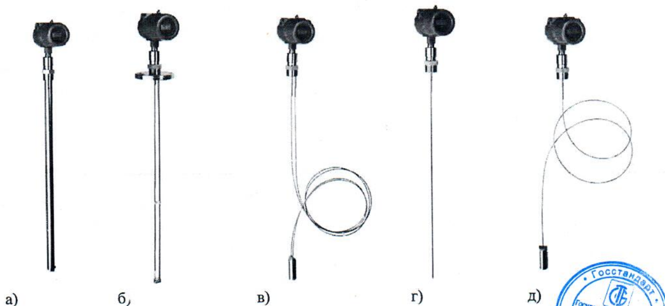
Рисунок 1 - Общий вид уровнемеров 3300 с различными типами волноводов (зондов):
