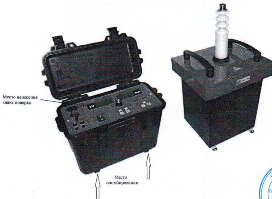
Рисунок 2 - Общий вид аппаратов испытания диэлектриков «АИД-70М» (модификация 2)
