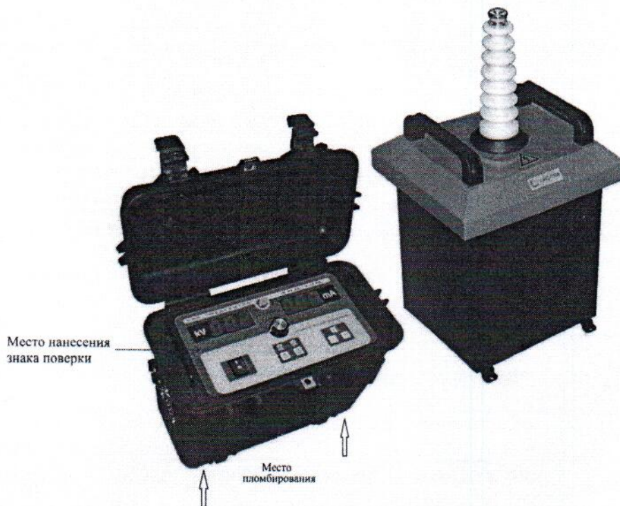
Рисунок 1 - Общий вид аппаратов испытания диэлектриков «АИД-70М» (модификация 1)
