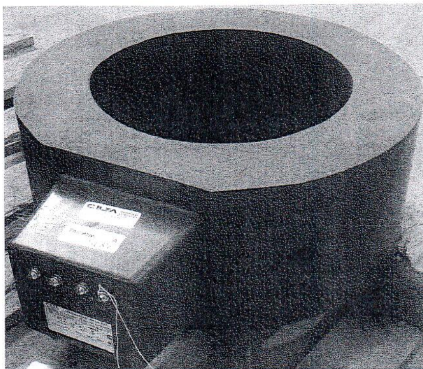
Рисунок 3 - Общий вид трансформаторов тока ТШЛ-СВЭЛ-20
