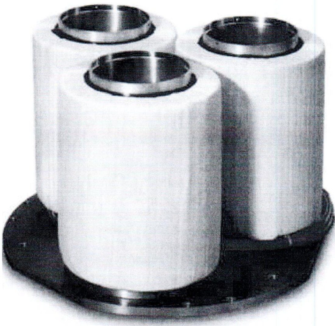
Рисунок 1 – Внешний вид трансформатора тока измерительного ELK-CT0.
